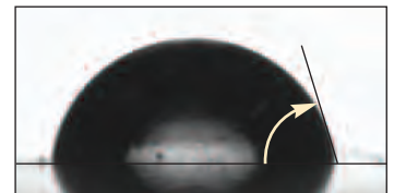
Eclipse für Coil nach Abriebtest: Kontaktwinkel = 84,1°
